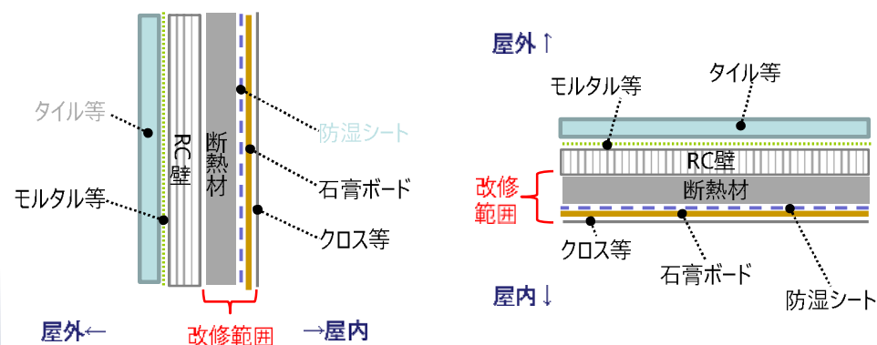
図2-5 横から見た断面図
