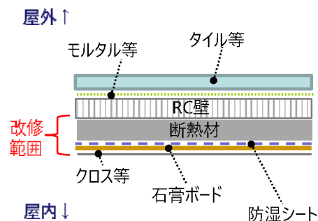
RC造(壁式構造・内断熱の場合)
